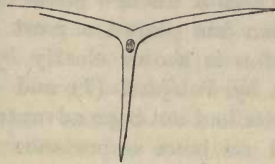
FIG. 9.—Alate spicule of L. Lieberkühni ( \times 150 ).
